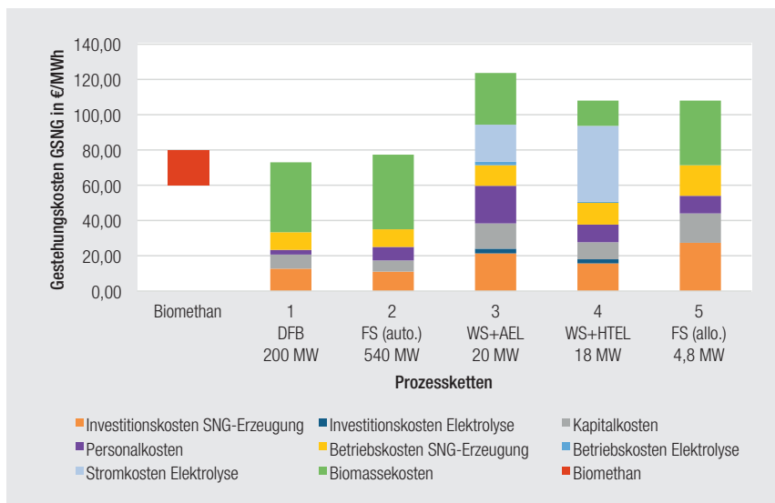
Abb. 6: SNG-Gestehungskosten (bezogen auf den Heizwert) der Prozessketten bei typischen Anlagengrößen und Biomethan als Benchmark (DFB: Dual Fluidized Bed, FS: Flugstrom, WS: Wirbelschicht, auto.: autotherm, allo.: allotherm, PEM: Proton Exchange Membrane Elektrolyse, AEL: Alkalische Elektrolyse, HTEL: Hochtemperaturelektrolyse)
