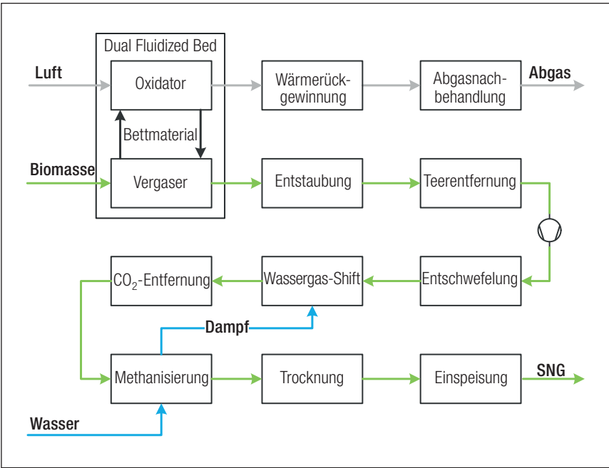
Abb. 5: Verfahrensschema der Referenzprozesskette 1
