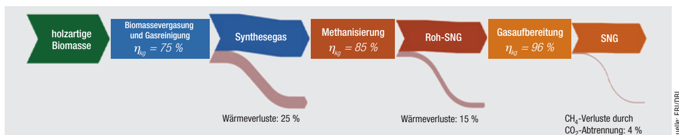
Abb. 1: Vereinfachtes Schaubild der Prozessstufen zur Erzeugung von SNG, nach [8] (Referenzprozesskette 1)
